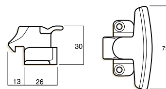
Non lockable
