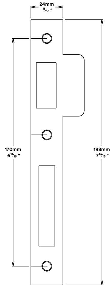
Striker Plate
